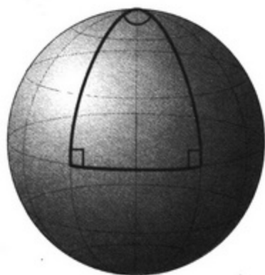
1.曲率为正
