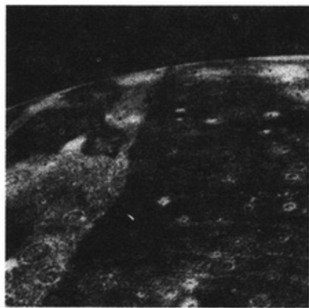
甘尼梅
