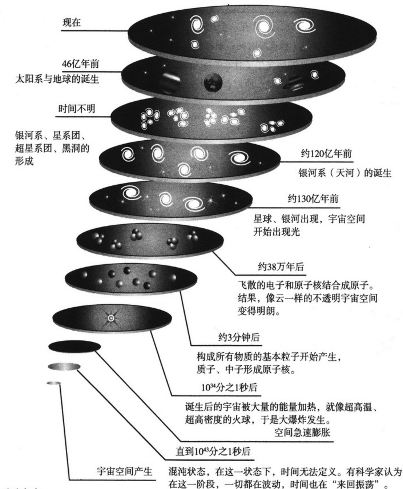
宇宙年表
