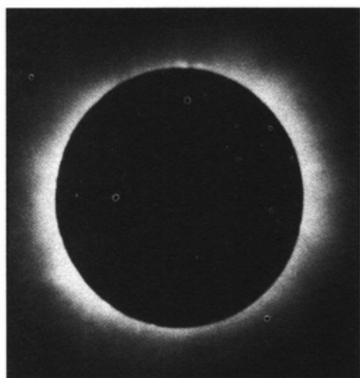
太阳的日冕
