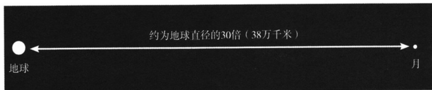
月球与地球距离比例图
