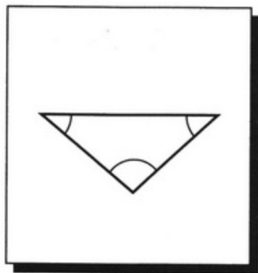
2.曲率为0
