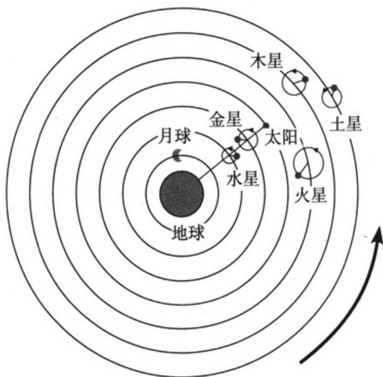
托勒密构想的天动说模型
