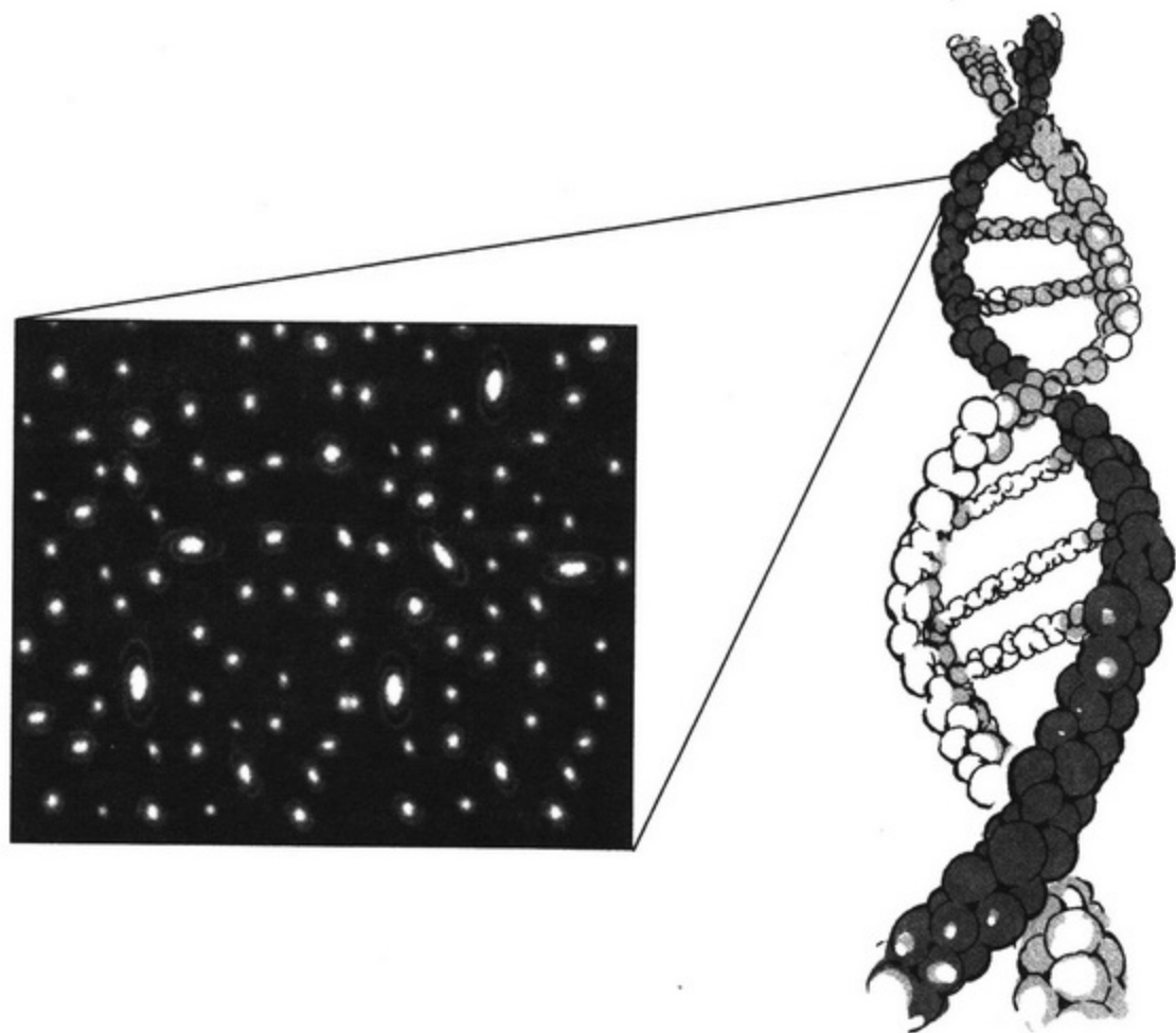
多元宇宙的假想图
