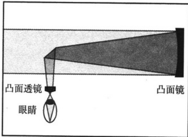
牛顿式望远镜
