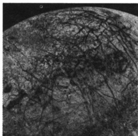
欧罗巴
