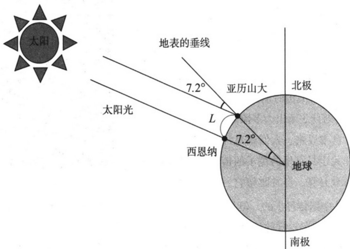
埃拉托色尼的计算方法
