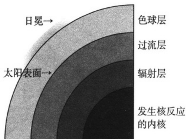
太阳的内部构造
