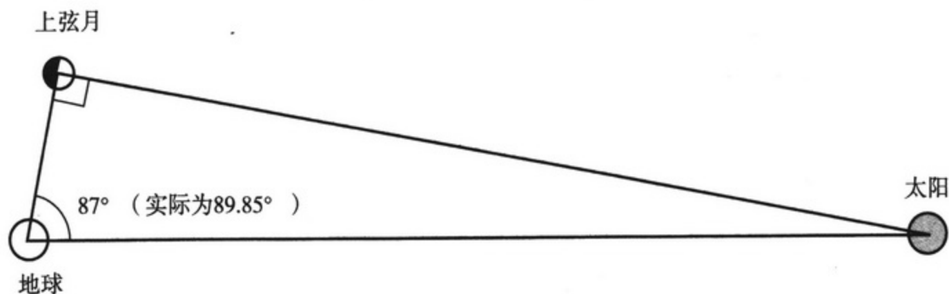
地球到太阳距离的计算
