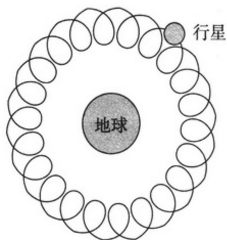
天动说中行星的运动2
