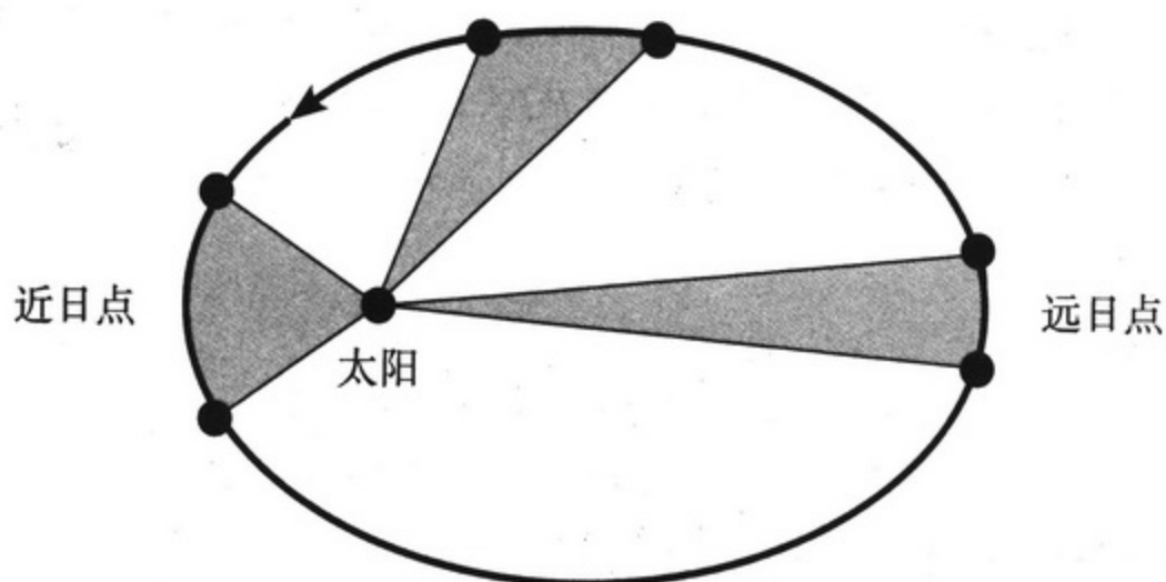
开普勒第二定律 行星的轨道1
