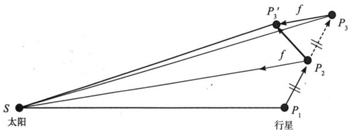
开普勒第二定律 行星的轨道2
