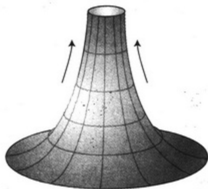
二维宇宙模型3
