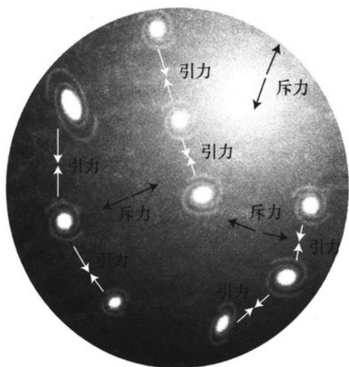
爱因斯坦考虑的静态宇宙模型
