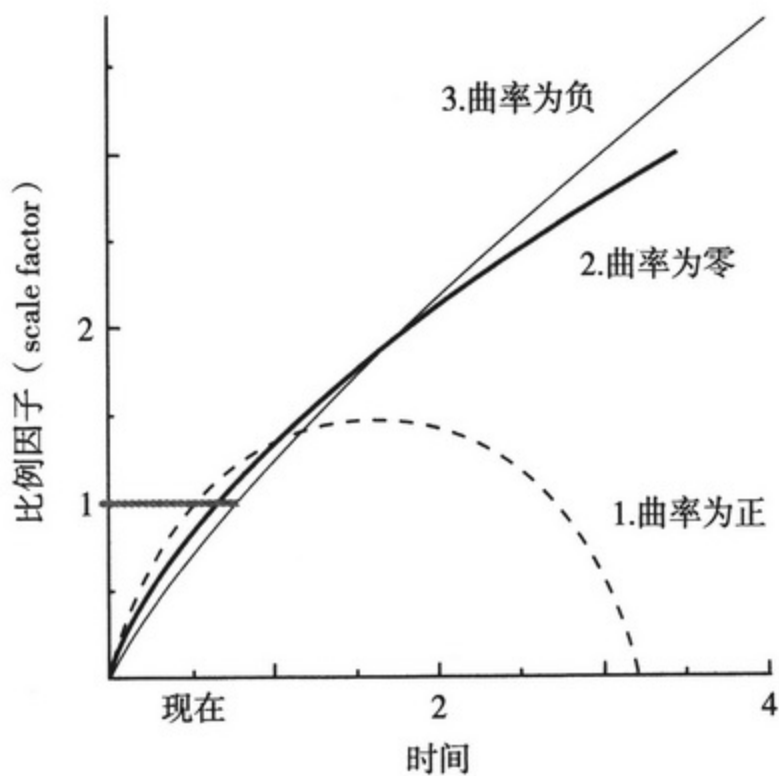
弗里德曼宇宙模型的时间变化
